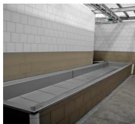
Ванна обескровливания, нержавеющая сталь, 8 м
