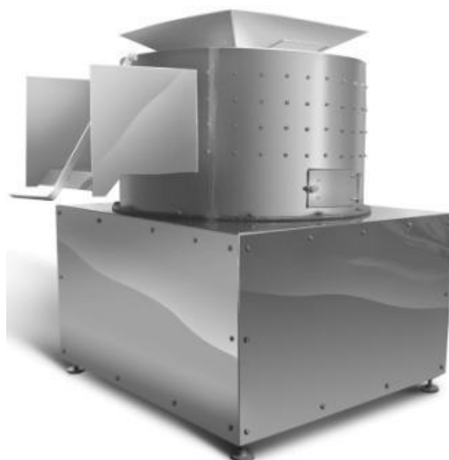
Очиститель центробежный для обработки слизистых субпродуктов
